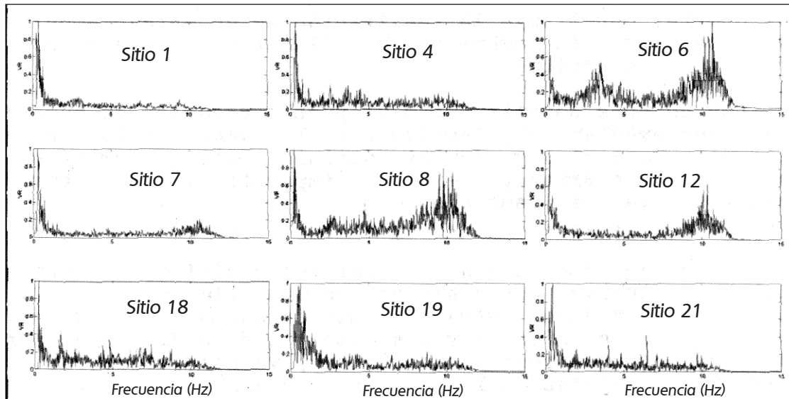
Figura 9. Espectros verticales promedio normalizados de algunos sitios de registro adquiridos en 2004. Se observa alta similitud en la forma y predominancia del pico entre 0.25 y 0.3 Hz.
