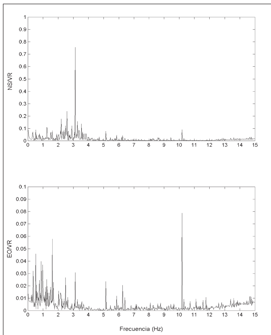
Figura 7. Cocientes espectrales obtenidos para el sitio 3.
