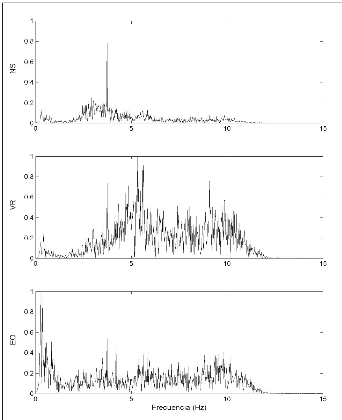
Figura 6. Espectros promedio normalizados, para cada dirección de movimiento, correspondientes al sitio 3.
