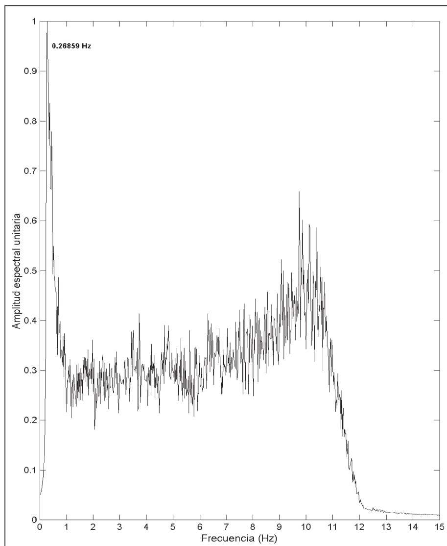
Figura 8. Espectro promedio vertical normalizado para Tuxtla Gutiérrez.
